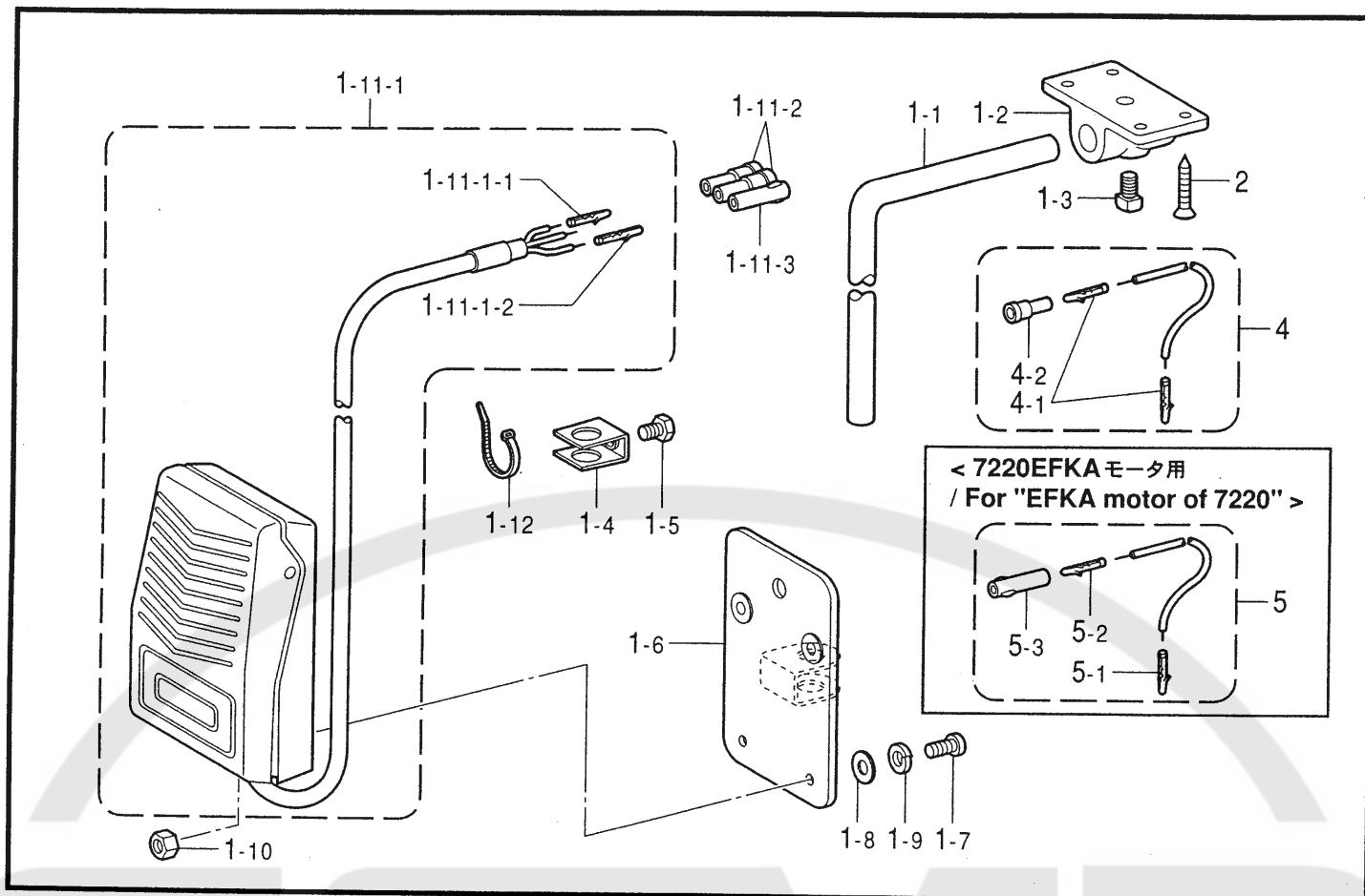
T. 逆転スイッチ関係 (7220, 7240) / Quick reverse switch mechanism (7220, 7240)
