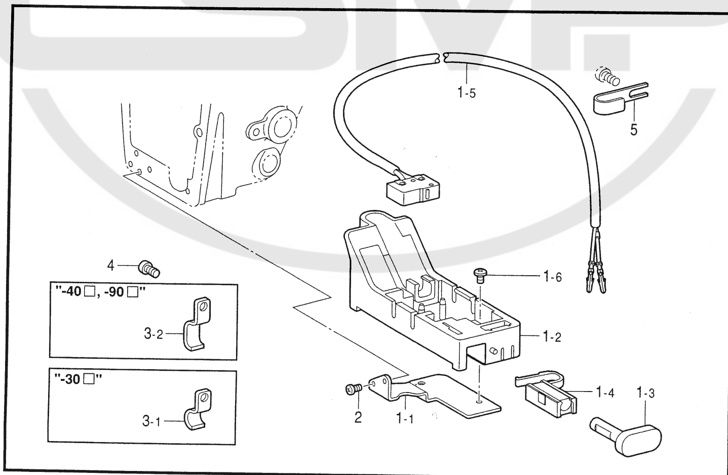
T. 逆転スイッチ関係 (7220, 7240) / Quick reverse switch mechanism (7220, 7240)
