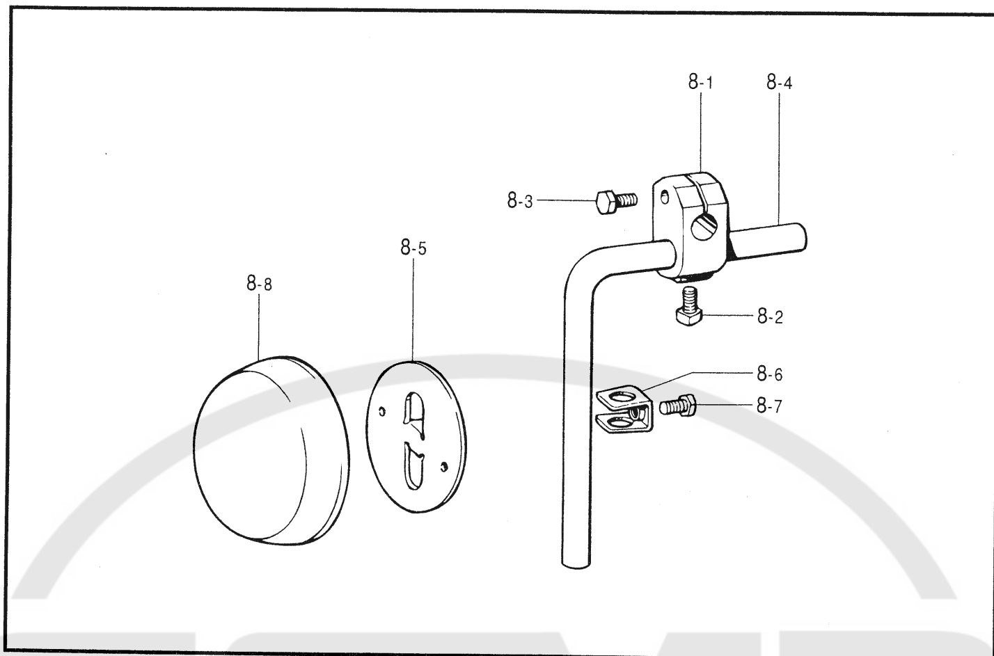
G. 逆転関係 (7220, 7240: -30□, -40□, -90□用) / Quick reverse mechanism (7220, 7240: -30□, -40□, -90□)
